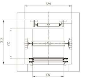
CWR (противовес сзади)
