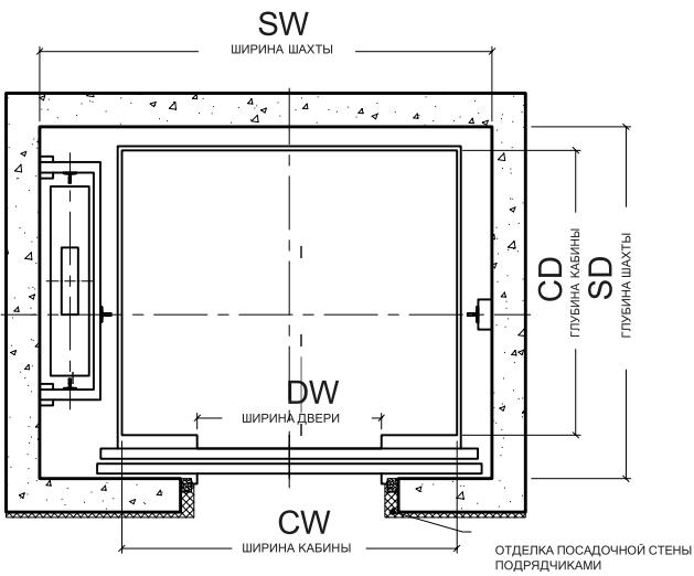
ШАХТА В ПЛАНЕ
