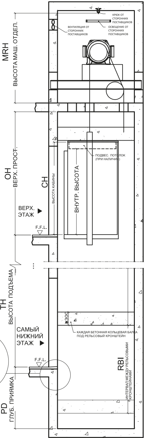
ШАХТА В РАЗРЕЗЕ
